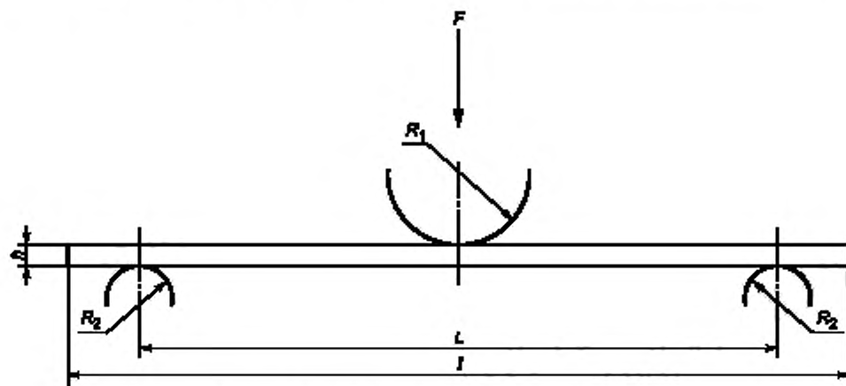
Рисунок ДА.1 — Схема трехточечного нагружения
