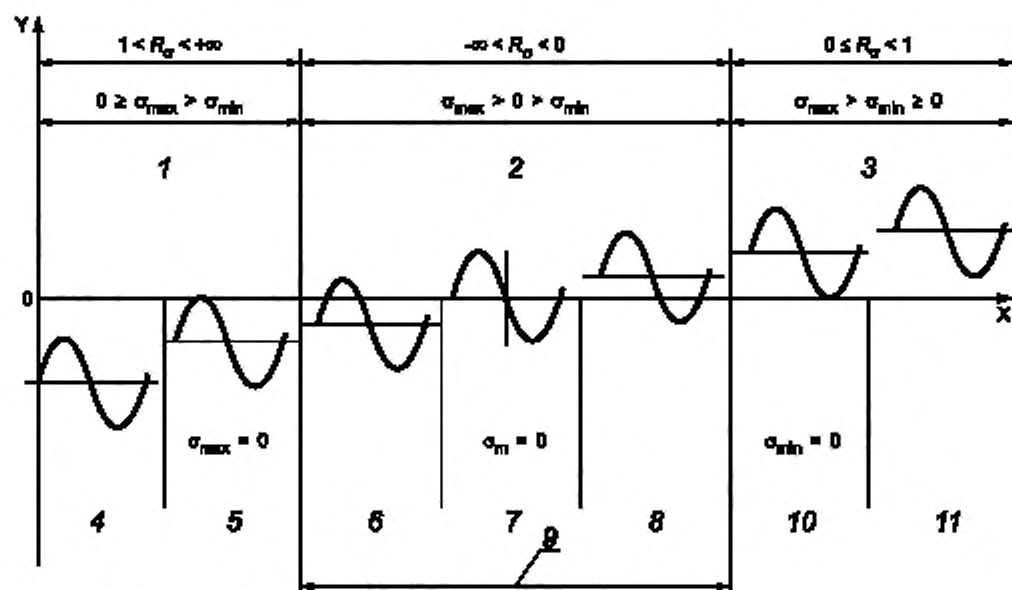
X — время t ; Y — напряжение \sigma (или деформация \epsilon ); 1 — область пульсирующего сжатия; 2 — область растяжения-сжатия; 3 — область пульсирующего растяжения; 4 — цикл пульсирующего сжатия, 5 — отнулевой цикл сжатия; 6 — знакопеременный цикл с преобладанием сжатия; 7 — симметричный или завершённый знакопеременный цикл; 8 — знакопеременный цикл с преобладанием растяжения, 9 — знакопеременные циклы; 10 — отнулевой цикл растяжения; 11 — цикл пульсирующего растяжения
