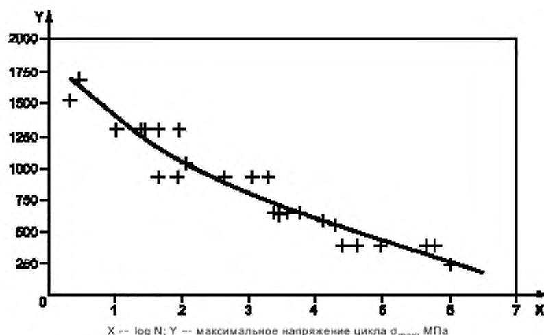
Рисунок 1 — Пример кривой усталости
