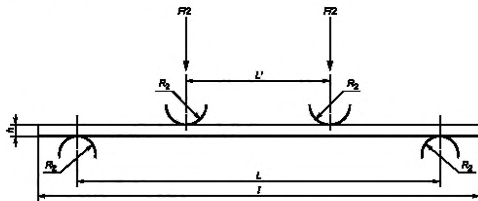
Рисунок ДА.2 — Схема четырехточечного нагружения
