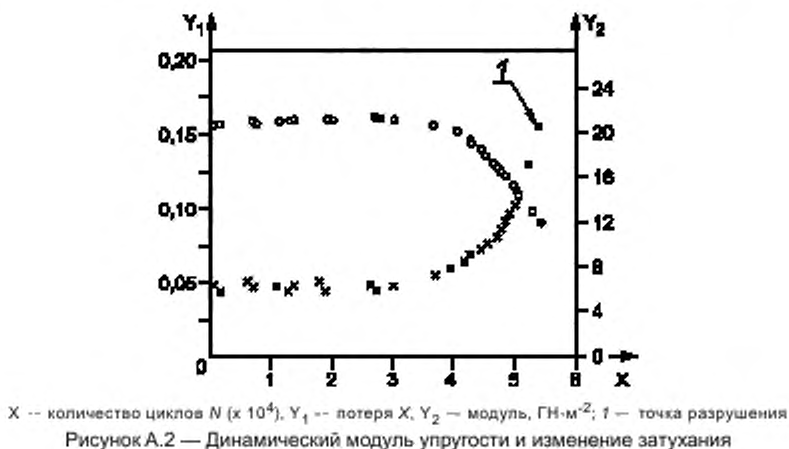
Рисунок А.2 — Динамический модуль упругости и изменение затухания
