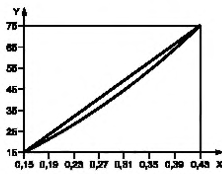
Рисунок В.1 — Типовая петля гистерезиса
