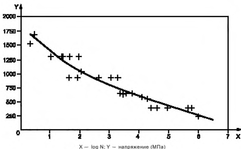
Рисунок 3 — Пример диаграммы усталости
