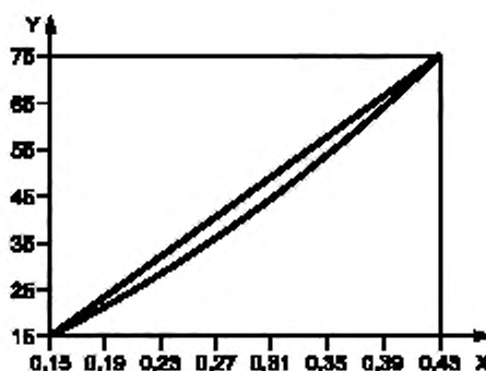
X — деформация, %; Y — напряжение, МН·м -2 Рисунок А.1 — Типовая петля гистерезиса
