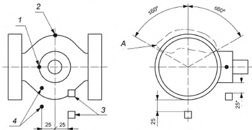
1 — термопара на крышке ИА; 2 — термопара на корпусе ИА; 3 — датчики температуры (кубы калориметра) пламени, 4 — термопара для измерения температуры пламени, А — участок, где устанавливают термопару корпуса. При установке в корпусе и крышке, термопары утапливают в корпус/крышку ИА на глубину \frac{1}{2} от толщины стенки или на 13 мм, в зависимости от того, какая величина меньше
