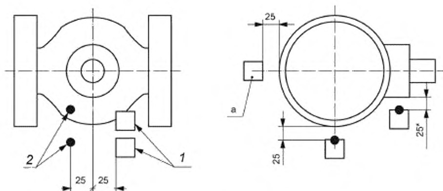
1 — датчики температуры (кубы калориметра); 2 — термопара для измерения температуры пламени, а — дополнительный датчик температуры (куб калориметра) для ИА DN ≥ 200
