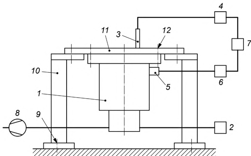
1 — турбомолекулярный насос; 2 — контроллер; 3 — датчик частоты вращения (например, фотодиод); 4 — устройство измерения частоты вращения; 5 — пусковое устройство; 6 — регулятор, пусковой механизм; 7 — регистратор данных; 8 — форвакуумный насос; 9 — анкерные болты; 10 — основание; 11 — опорная плита; 12 — установочные крепежные болты для насоса
